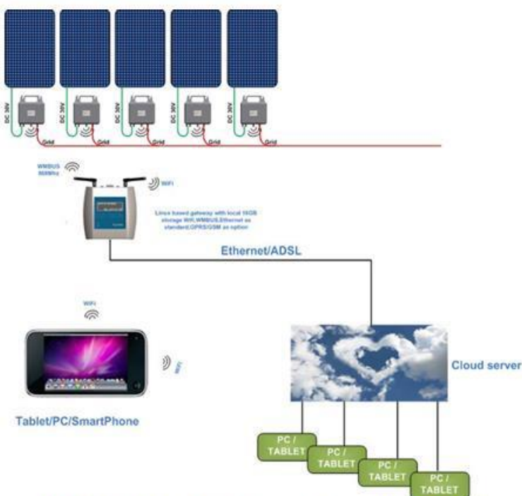
Slika 3: Podatkovna mreža za sončno energijo - struktura
